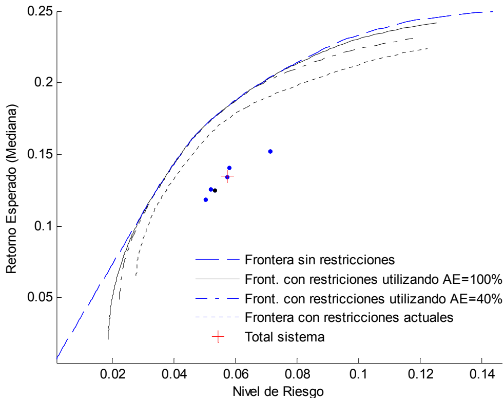
Figura 4. Fronteras eficientes con cambios en el límite de inversión en activos externos (AE). Retornos en UVR. Retornos esperados corresponden a las medianas históricas. Mayo de 2005.
