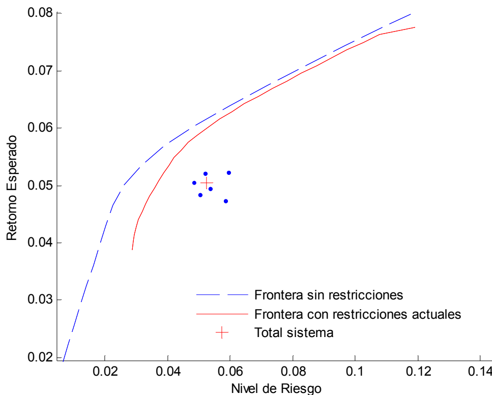
Figura 5. Eficientes con y sin restricciones. Retornos en UVR. Julio de 2004.
