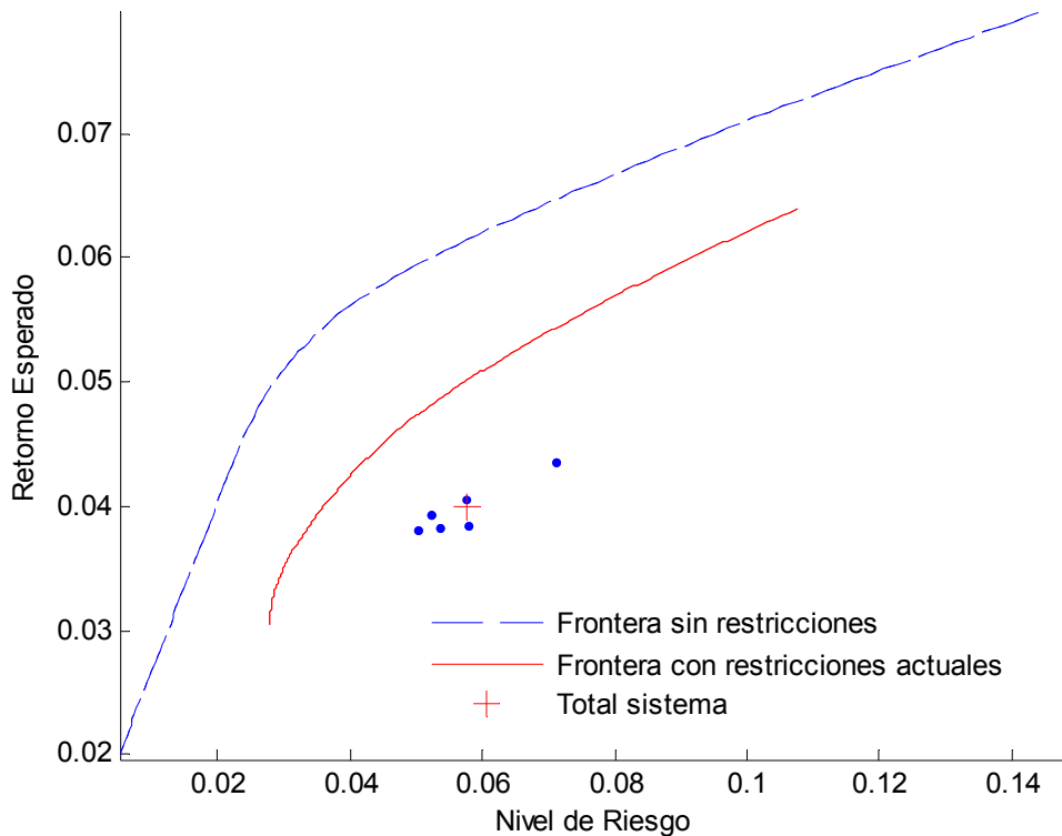
Figura 2. Fronteras Eficientes con y sin restricciones. Retornos en UVR. Mayo de 2005.
