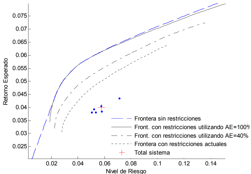
Figura 3. Fronteras eficientes con cambios en el límite de inversión en activos externos (AE). Retornos en UVR . Mayo de 2005.
