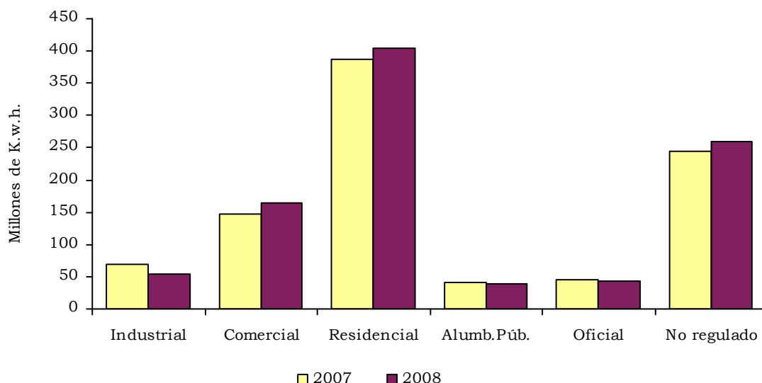
Gráfico 2.8.10.1.1 Tolima. Consumo de energía eléctrica, según usos. Acumulado enero a diciembre 2007 – 2008
