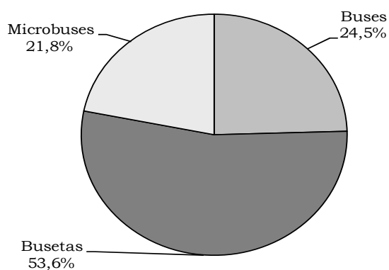
Gráfico 2.8.7.2. Área metropolitana de Bucaramanga. Distribución promedio diario en servicio 2009
