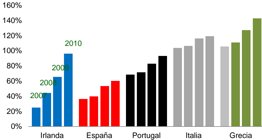
Deuda como porcentaje del PIB (2007-2010)
