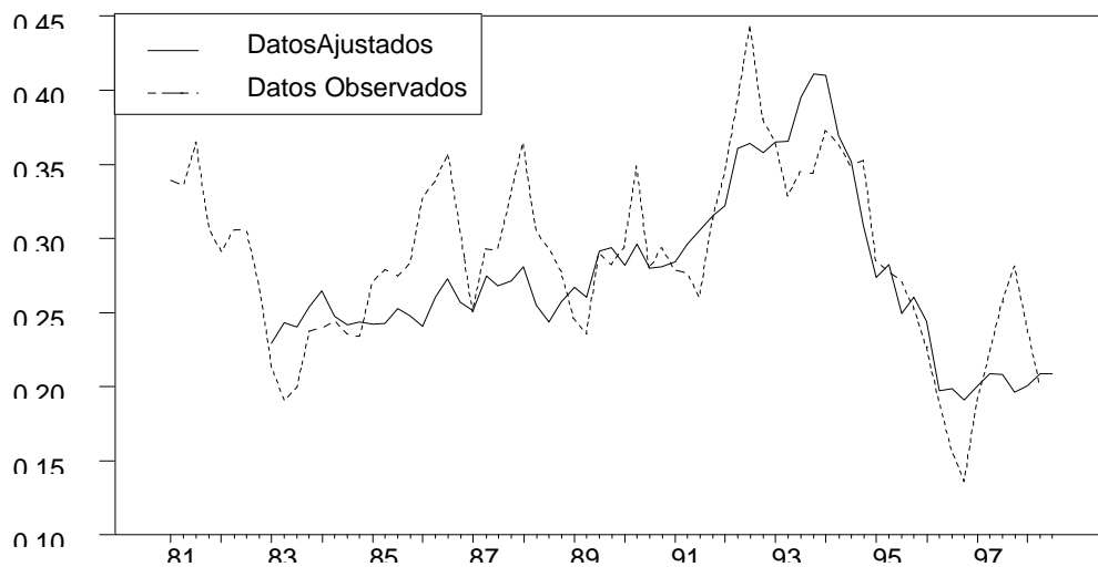
Gráfico 2 : Ajuste del modelo de demanda por base monetaria.
