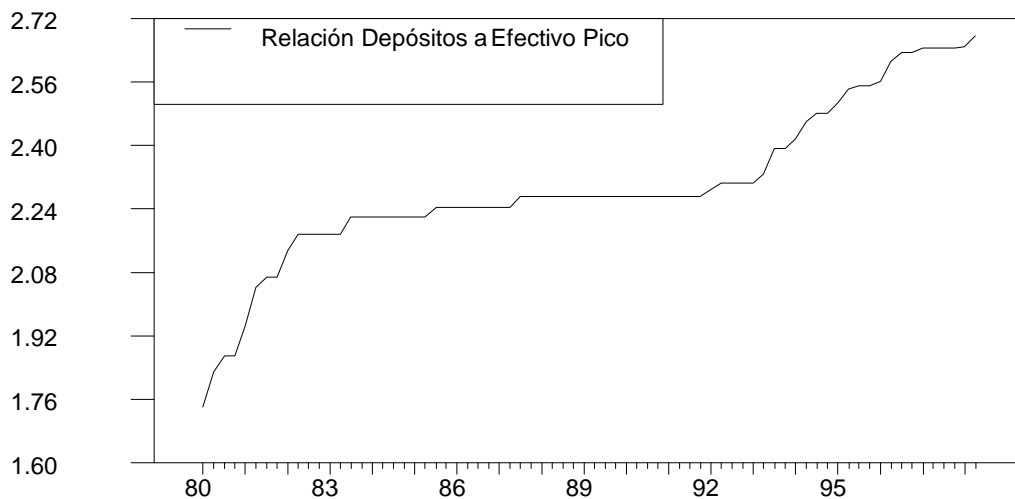
Gráfico 1 : Relación depósitos a efectivo pico.
