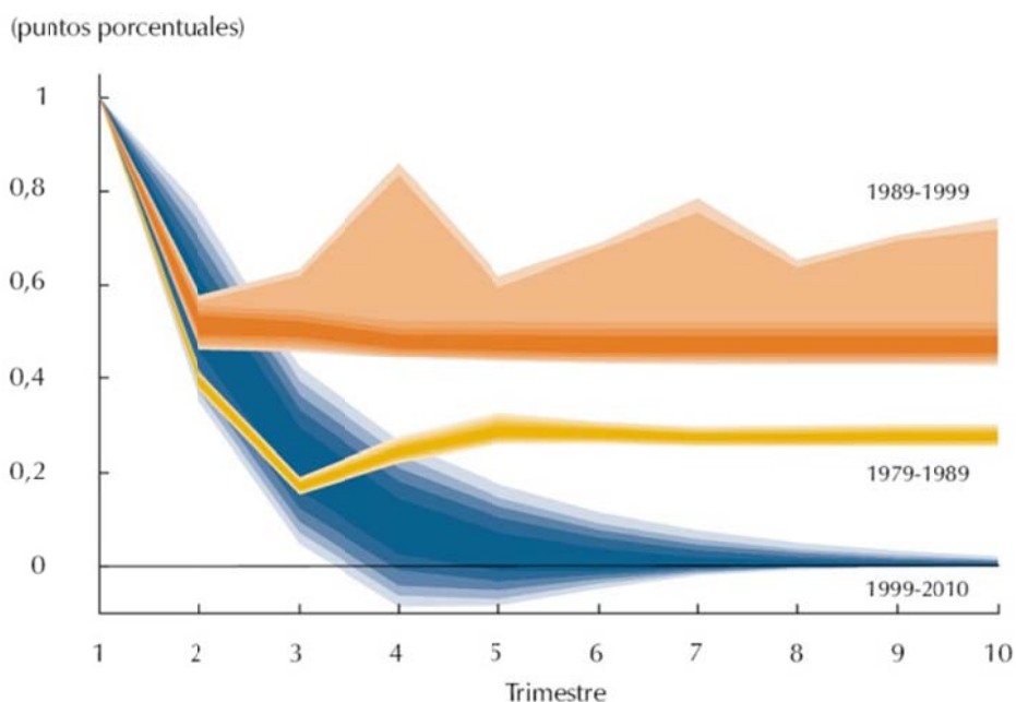
Gráfico 3 Funciones Impulso Respuesta en los 3 Regímenes
